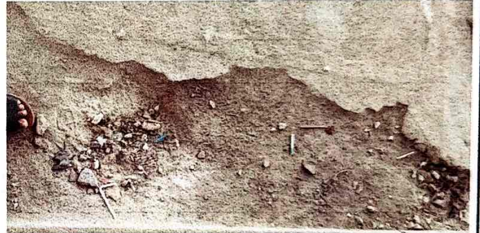
Foto 4: Reparación de entortado por deterioro, frente a la Dirección
